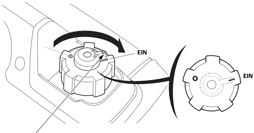
TANKDECKEL-LÜFTUNGHEBEL
