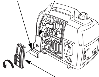
LUFTFILTERDECKEL
