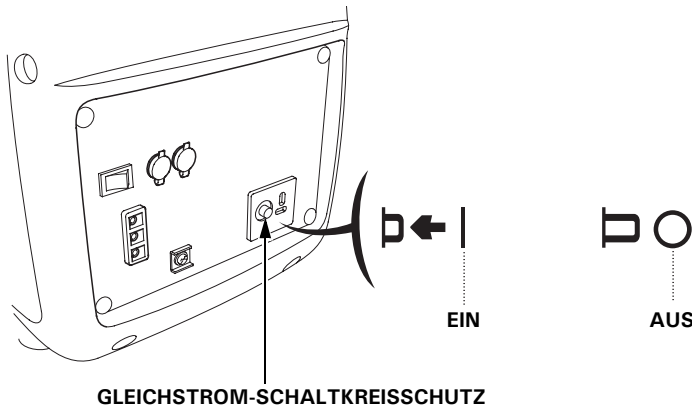
GLEICHSTROM-SCHALTKREISSCHUTZ
