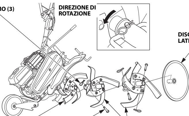
FRESA INTERNA LATO SINISTRO
