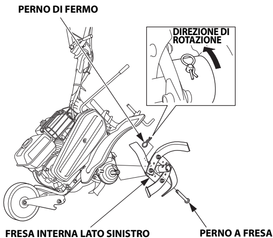
PERNO A FRESA (LUNGO)
