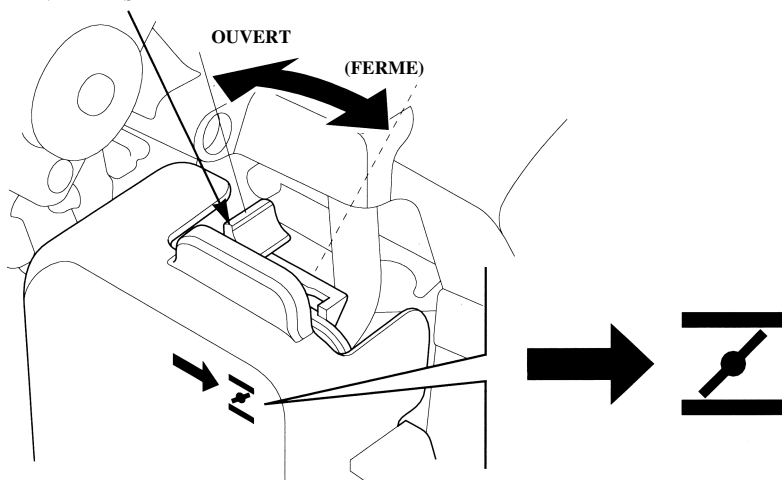
LEVIER DE STARTER
