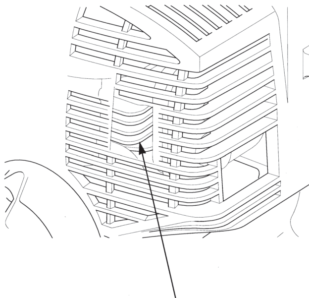
ALETTE DI RAFFREDDAMENTO (all'interno del coperchio)
